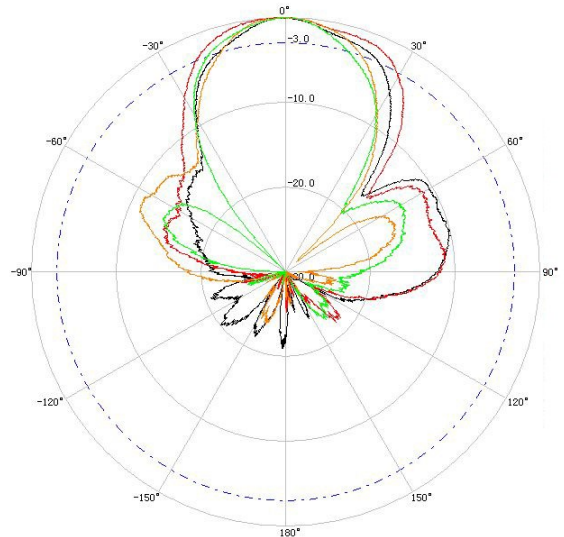
H-Plane
